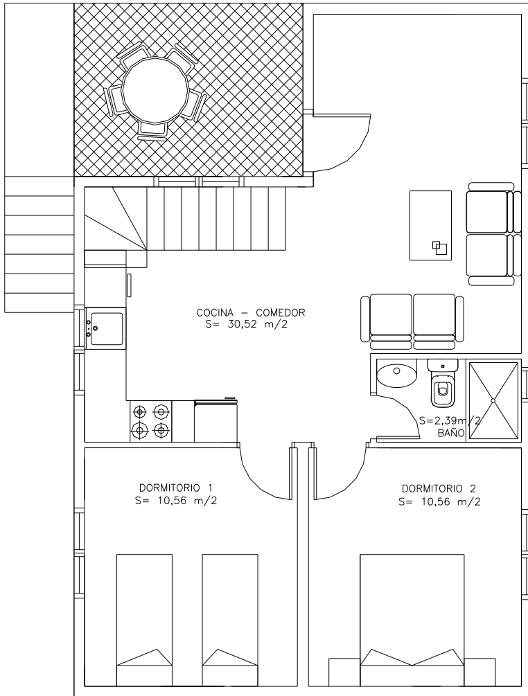
PLANTA PRIMERA
